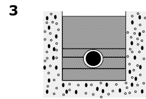
3 Verfüllen einer Lage bis 0.2 Meter über dem Rohrscheitel. Verdichten mit leichten Vibrationsmaschinen (nicht unmittelbar über dem Rohr).
